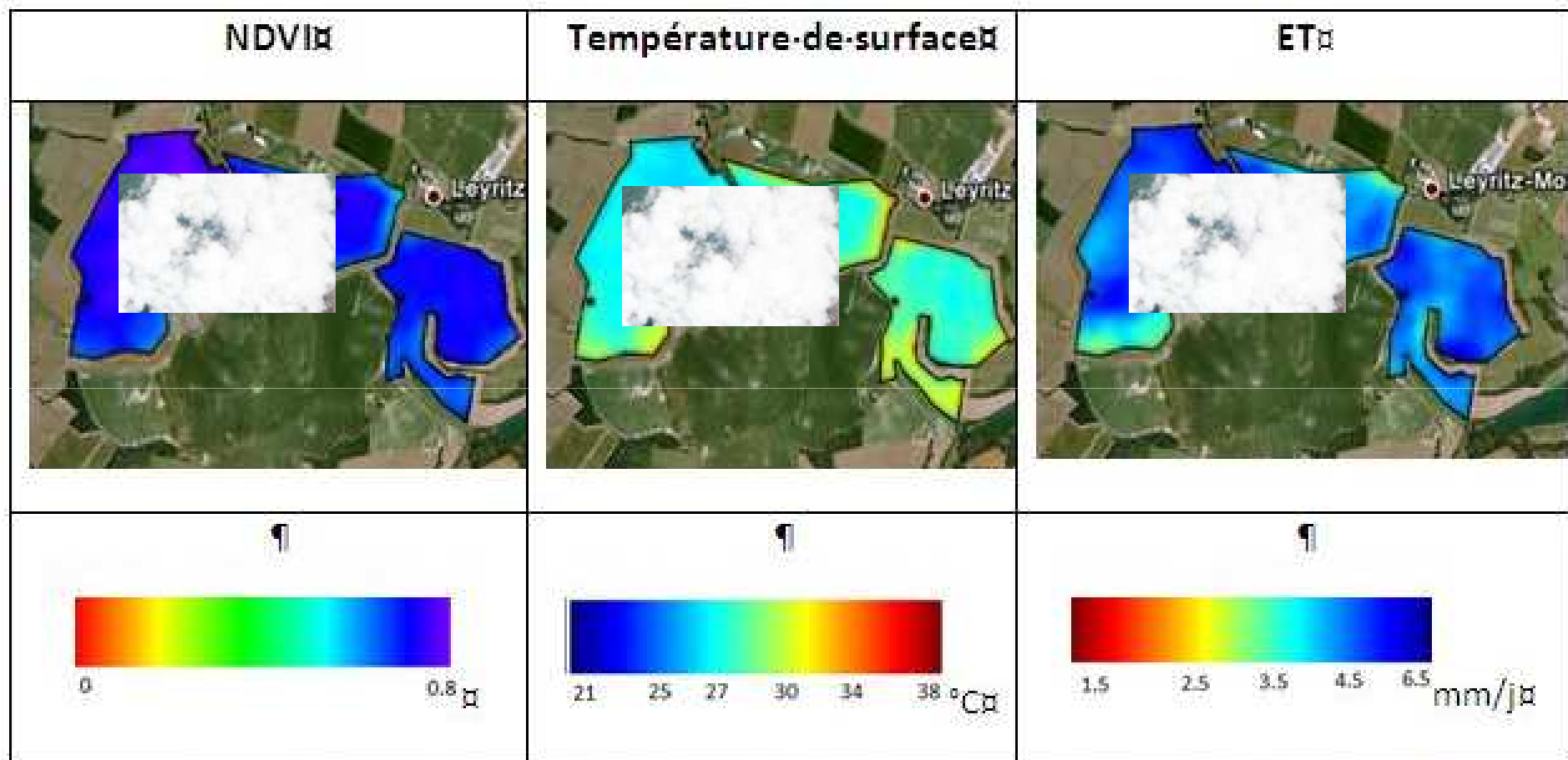
Figure-31:-Traitement-SEBAL-au-12-août-2011-sur-des-parcelles-de-mais(Château)¶
